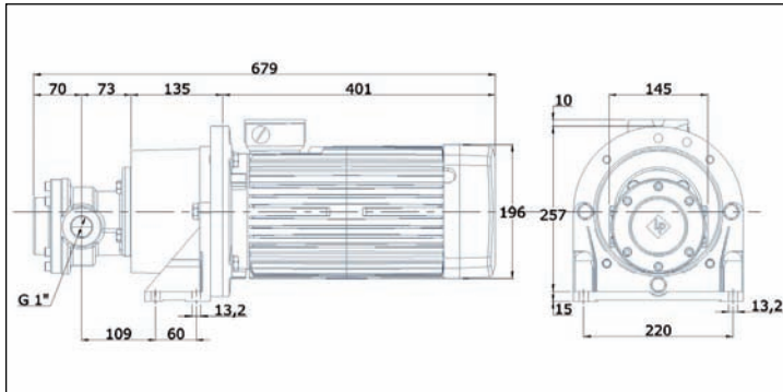
FOM 430- FOM 438 7,5 kW weight: 63,5 kg
