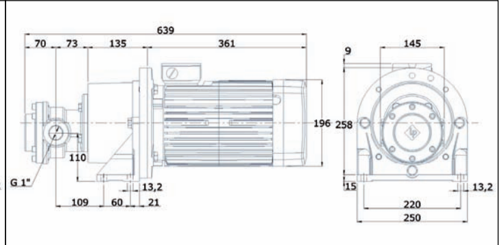
FOM 422- FOM 438 5,5 kW weight: 55,5 kg
