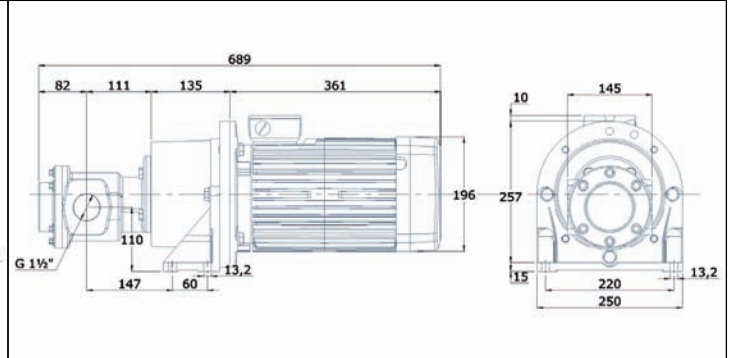
FOM 570- FOM 590 5,5 kW weight: 60 kg
