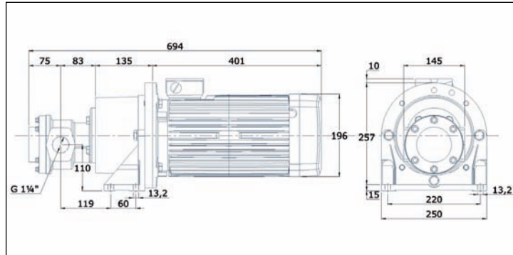
FOM 545- FOM 556 7,5 kW weight: 65 kg
