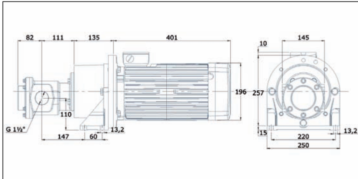
FOM 570- FOM 590 7,5 kW weight: 68 kg
