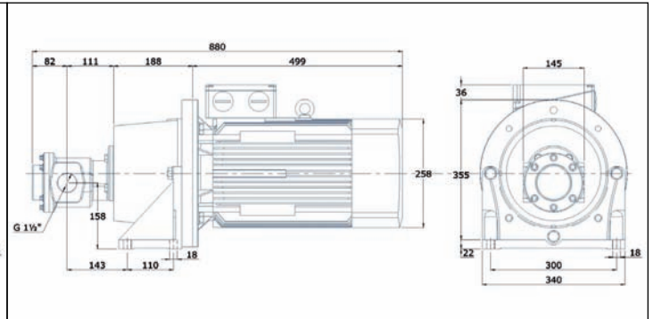
FOM 570- FOM 590 18,5 kW weight: 135 kg
